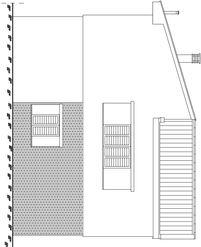
PROSPETTO 4-4
